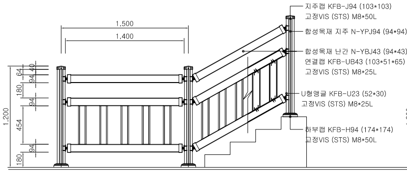
난간 입면도
