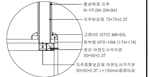
하부 접합 상세도
