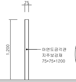
지주 보강재 상세도
