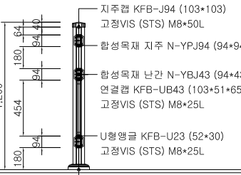
난간 단면도
